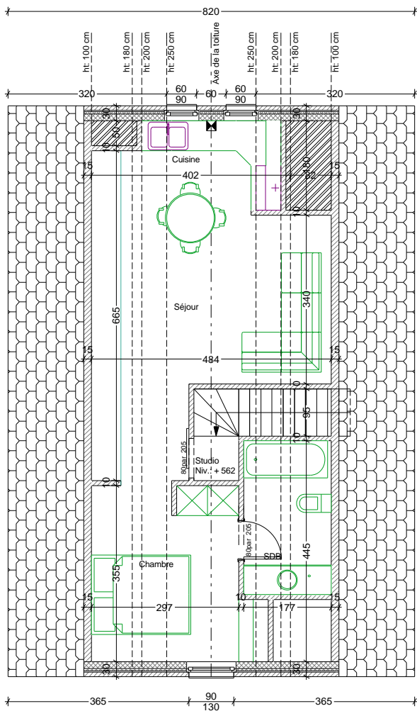
Vue en plan des combles aménagés
