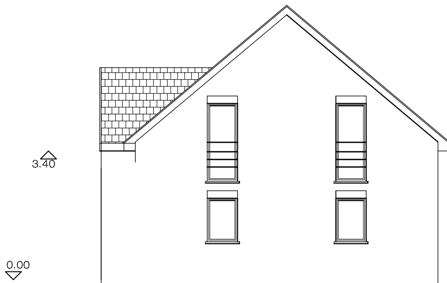
PIGNON DROIT
